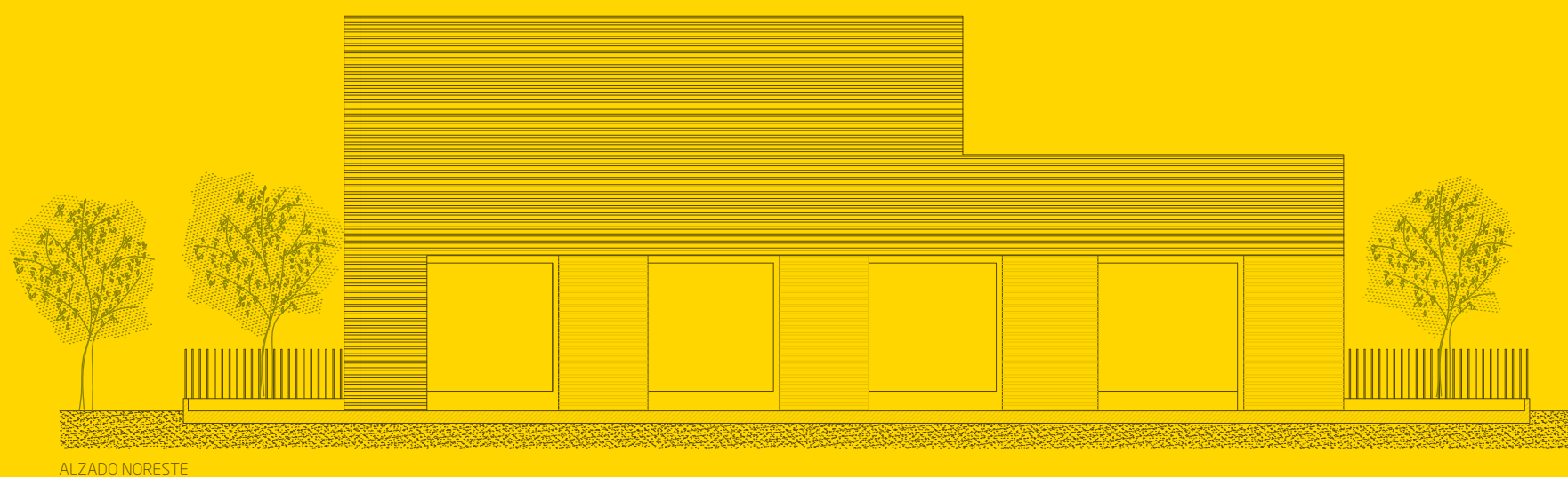
ALZADO NORESTE
